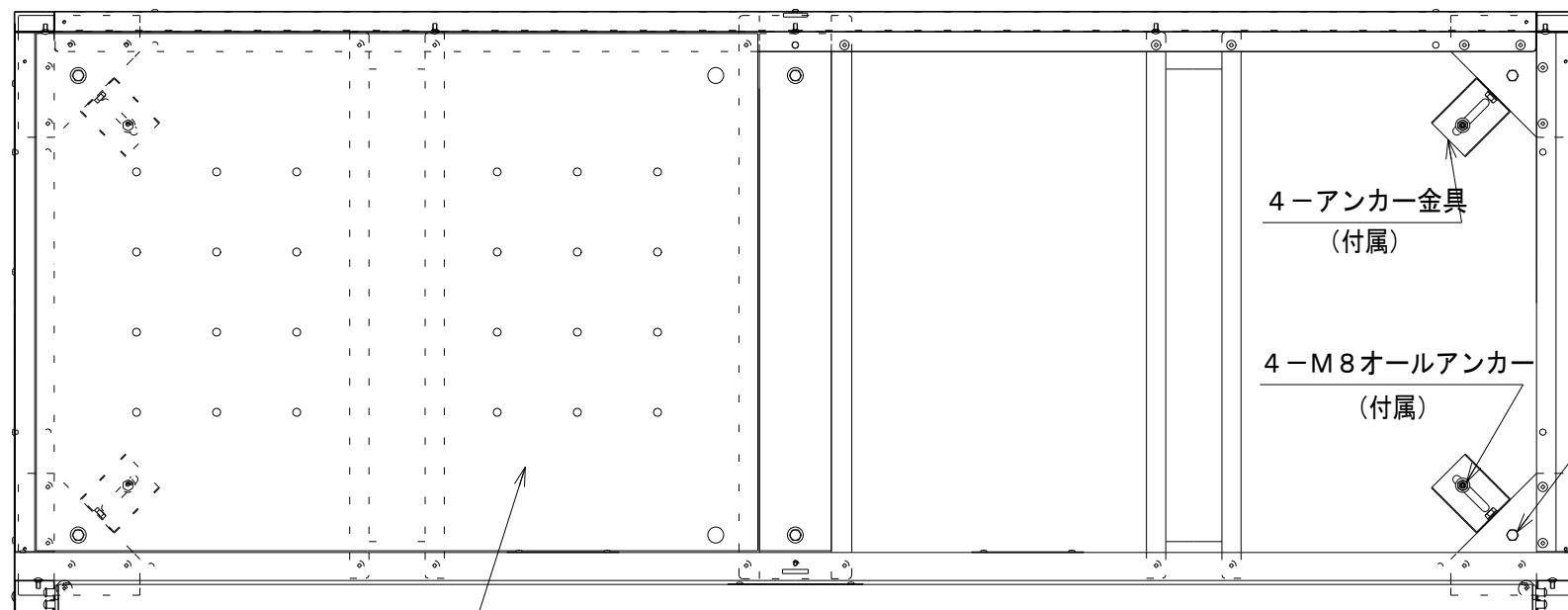
A-A断面図 (右底板を取り外した状態) 2-底板 (取り外し可能)
